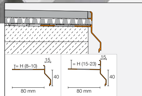
Montaż Schlüter®-BARA-RKKE
