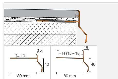
Montaż Schlüter®-BARA-RKK
